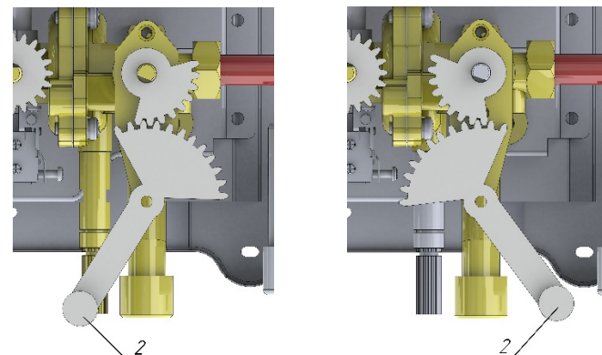
в) Рычаг управления регулятором расхода воды 2 в положении «Максимальный расход»
